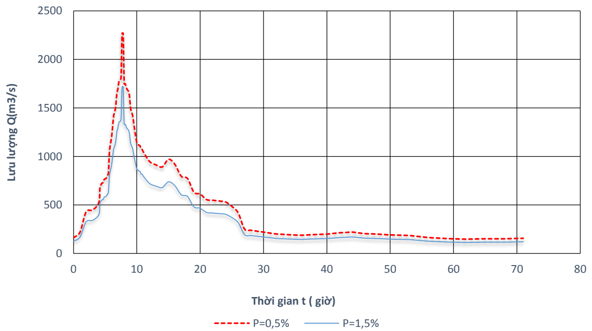
Biểu đồ tần suất lũ thiết kế tuyến đập Nậm Công 5
