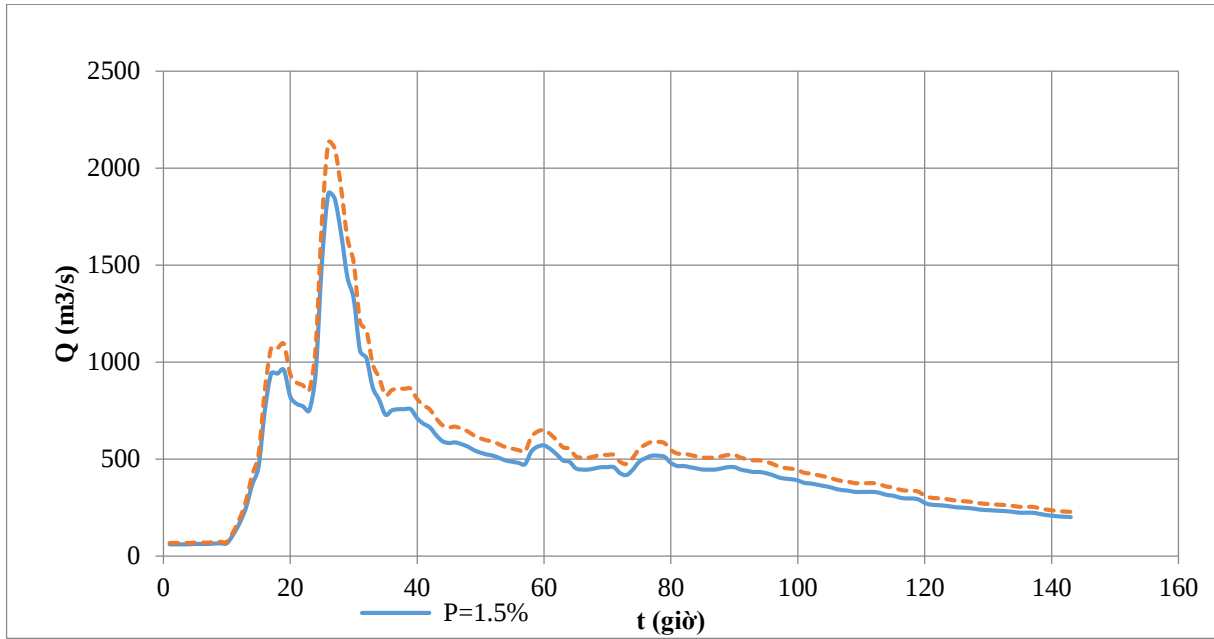
Phụ lục 5: Biểu đồ tần suất lũ công trình thủy điện Chiềng Công 1
