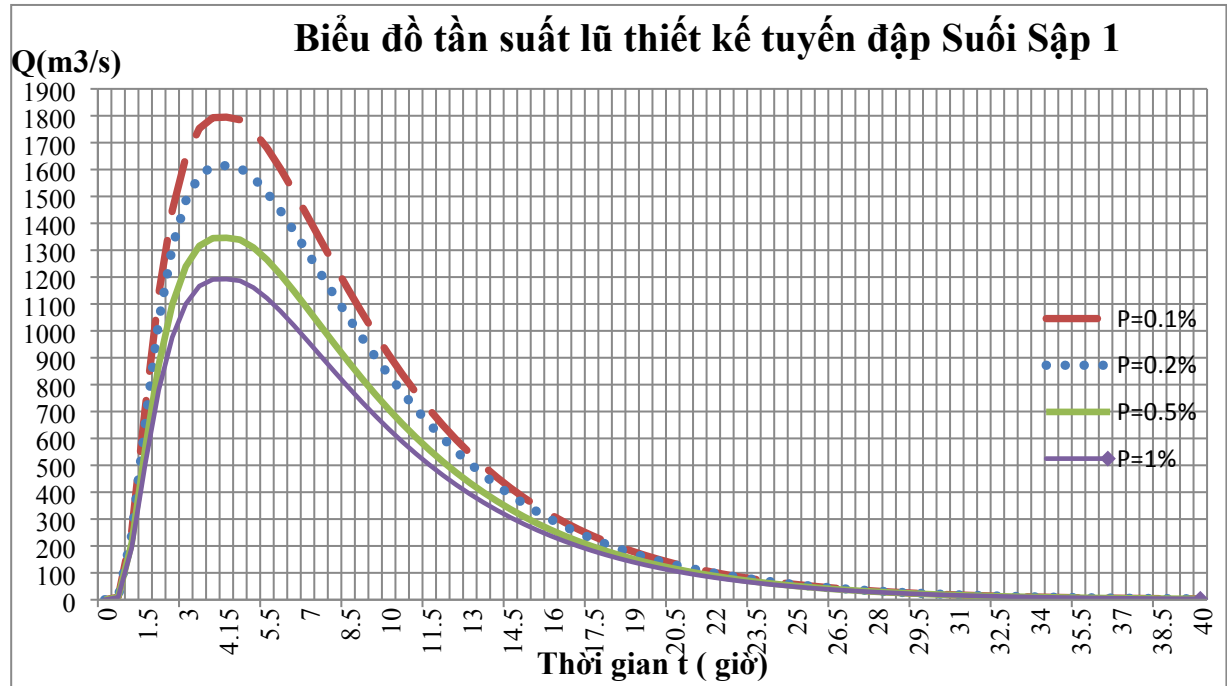
Phụ lục 5 : Biểu đồ tần suất lũ thiết kế Suối Sập 1
